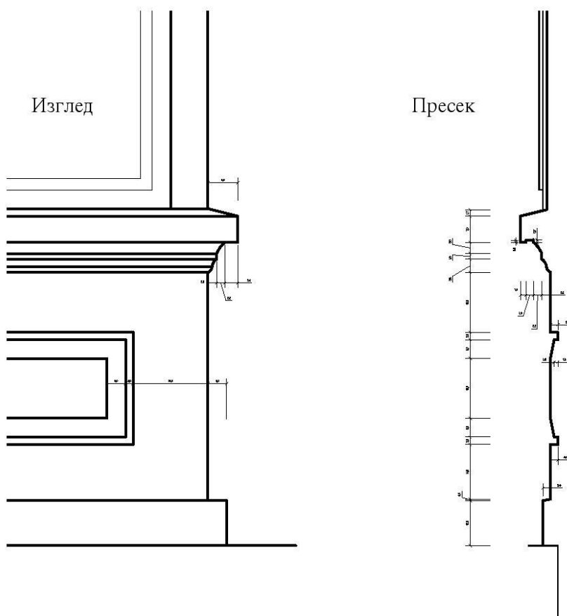
Профил 4 и 5
