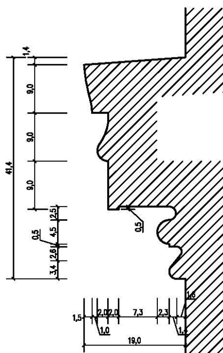
Пресек
