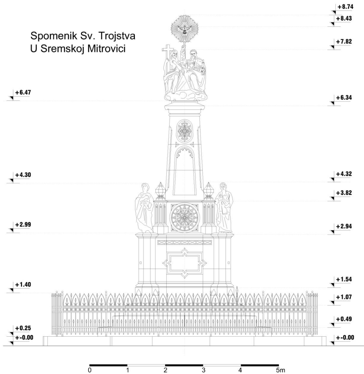
Izgled severo zapadni Projektovano stanje
