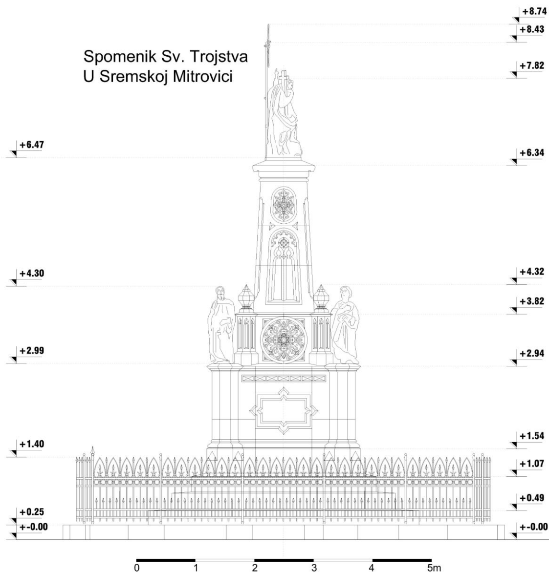
Izgled severo istočni Projektovano stanje
