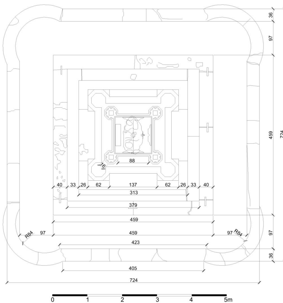
Osnova Postojeće stanje
