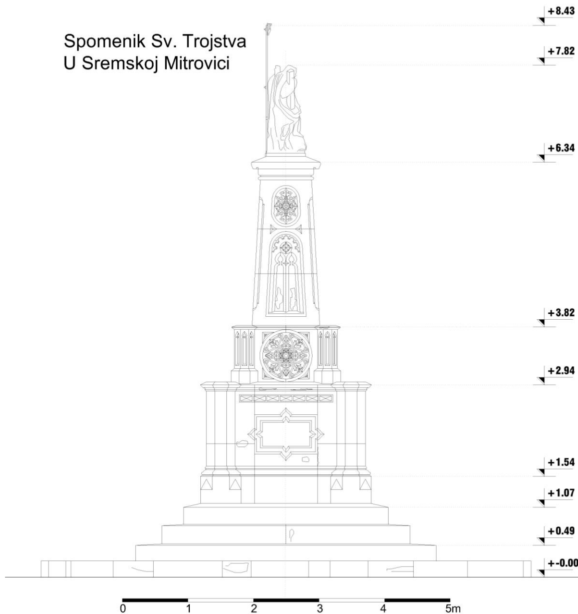
Izgled severo istočni Postojeće stanje
